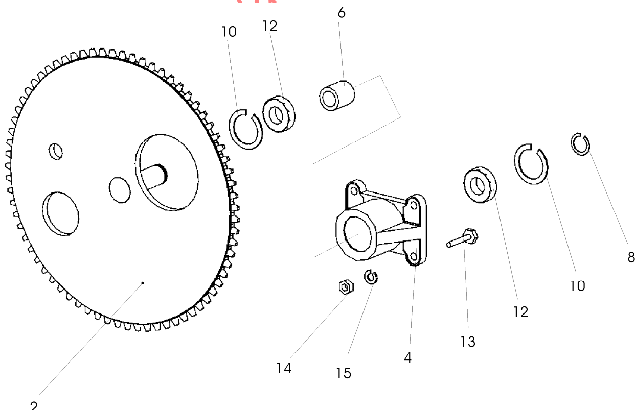
Рис. 14 ОВИ 02.250. Привод
