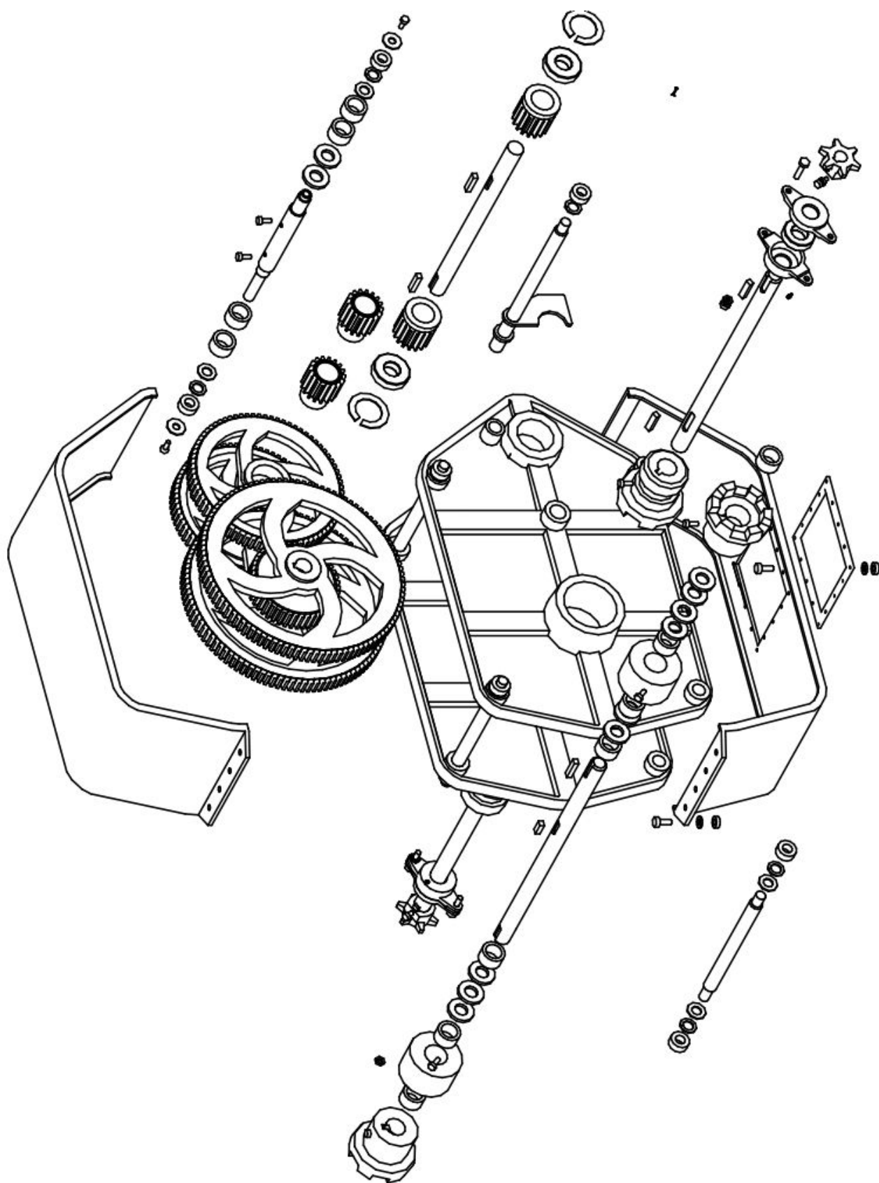
Рис. 29 ОВИ 06.100 Редуктор
