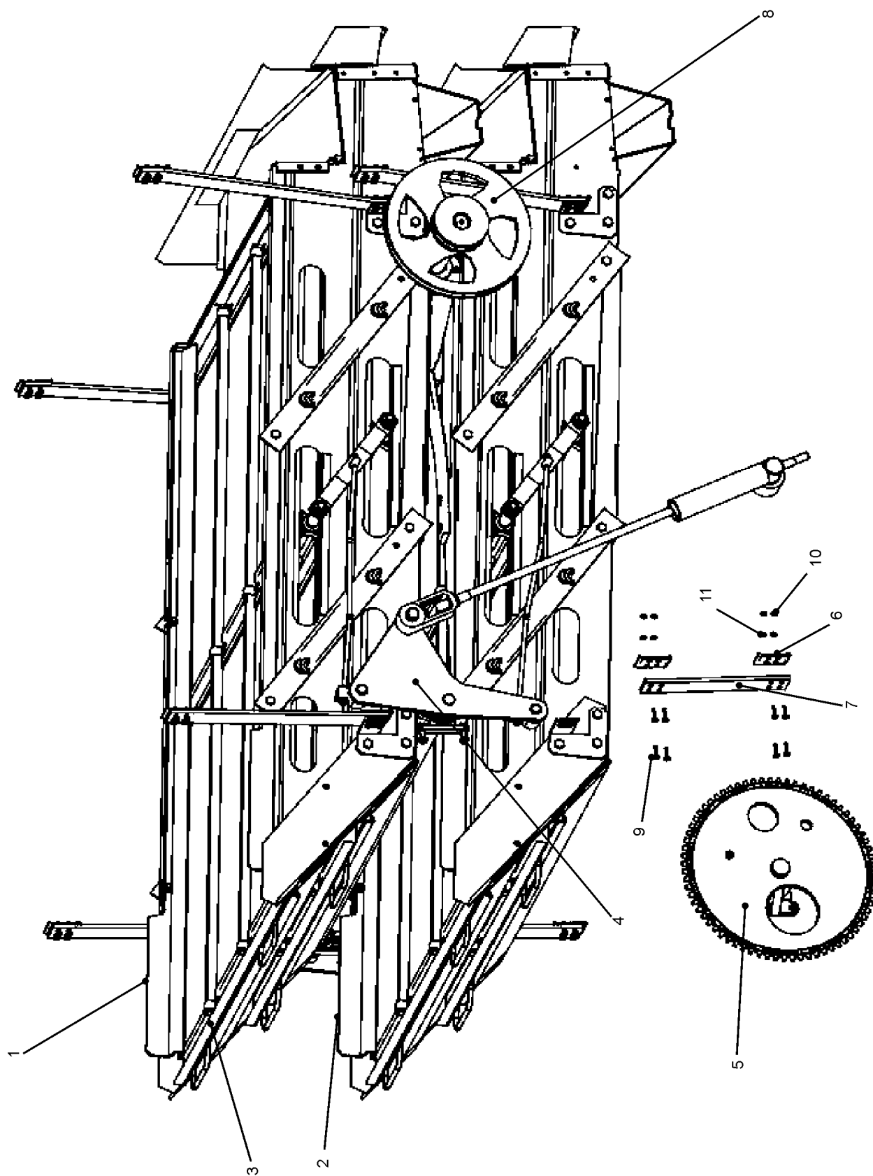
Рис. 7 ОВИ 02.000 Часть решетчатая
