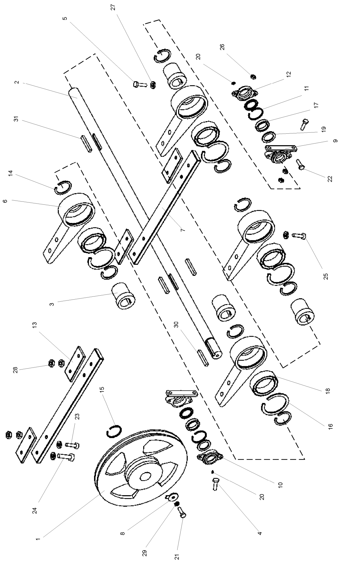
Рис. 11 ОВИ 02.140 Вал эксцентриковый
